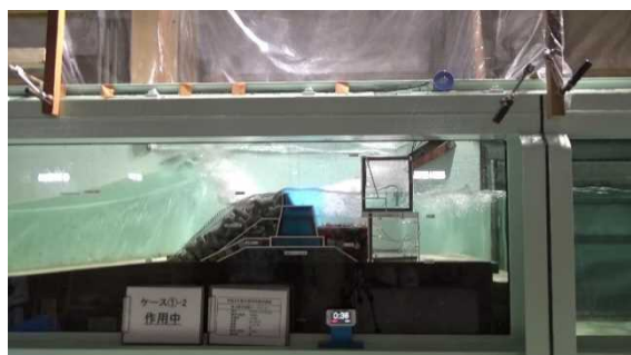
長水路における実験イメージ
