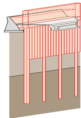
大分港海岸「楕形鋼矢板壁工法」
